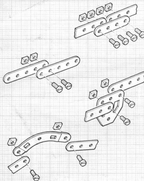
Esempi di giunzione - Exemples de jonction - Joints - Verbindungsbeispiele - Ejemplos de juntas.
