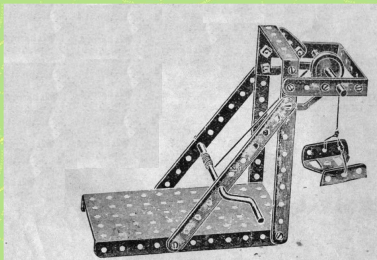
Fig. 34 - Bilancia a sospensione
